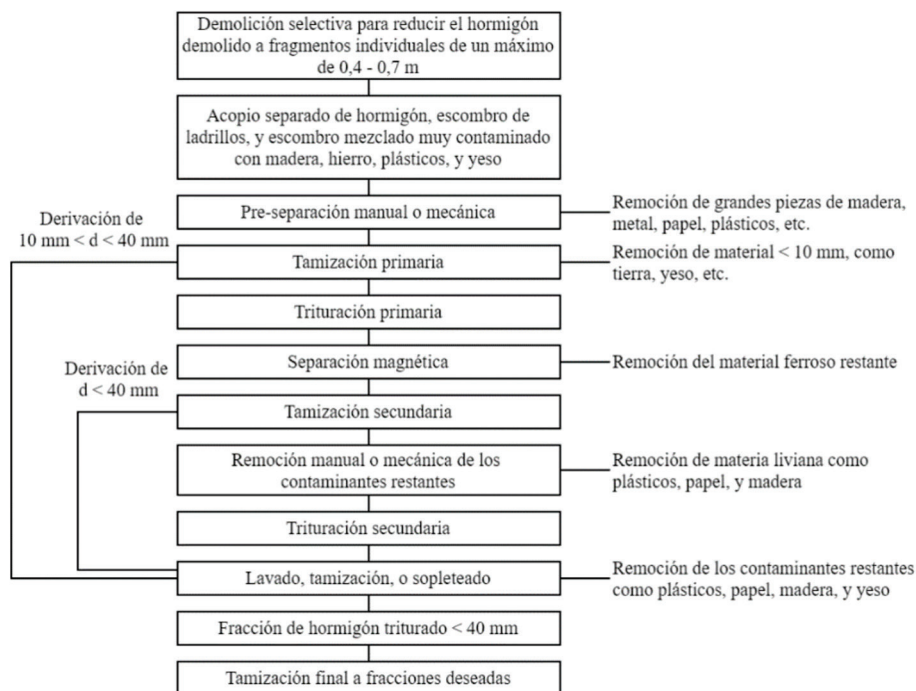
Figura 3: Planta de procesamiento de hormigón de demolición (adaptado de [19]).
