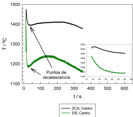
Figura 3: Curvas de enfriamiento en ZPA y VD ampliadas.
