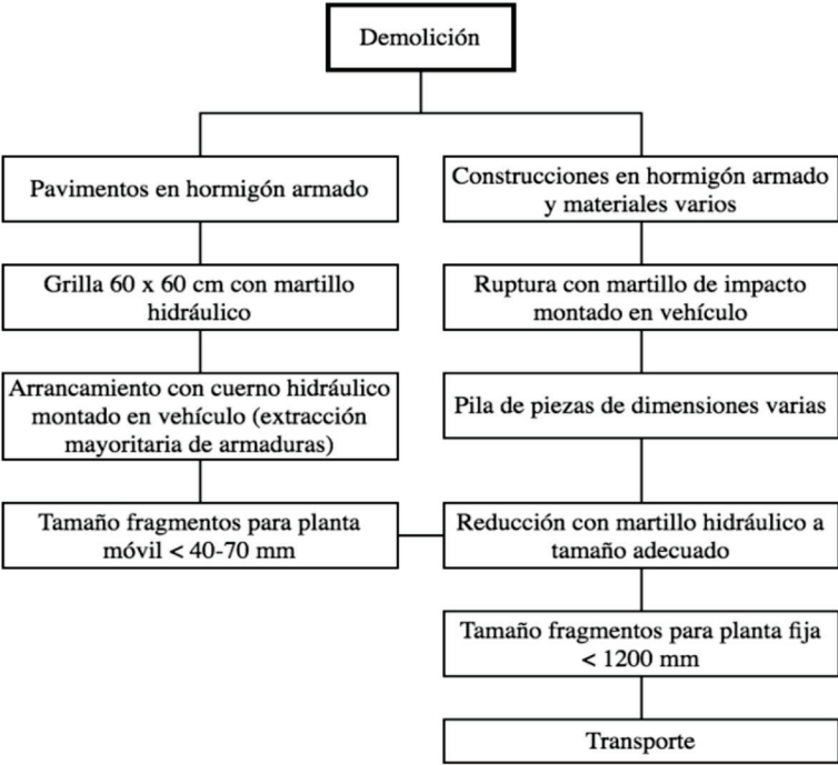
Figura 2: Esquemas de demolición, elaboración propia según reporte ACI-555-01 [19].
